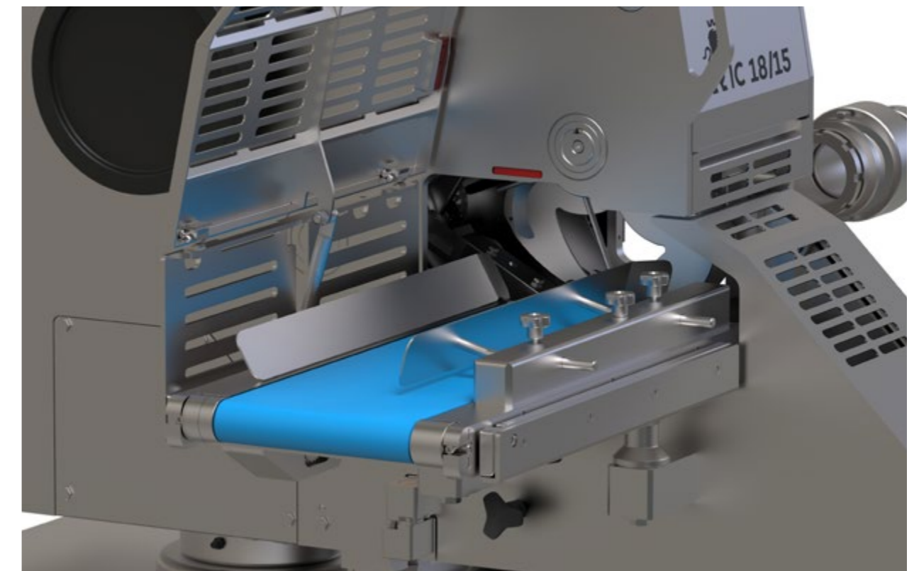
Pneumatic belt FDA certified / Nastro uscita prodotti certificato FDA
